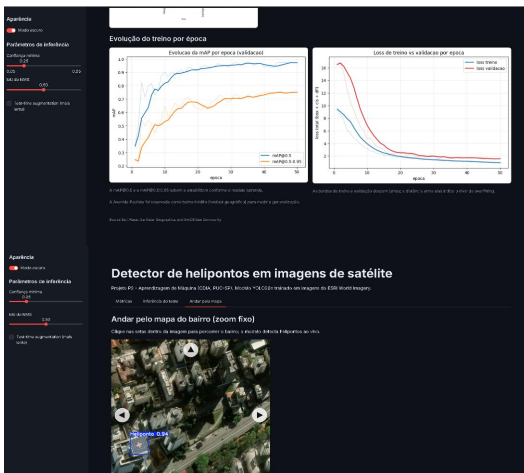
Figuras 9 e 10 - Telas da aplicação Streamlit
