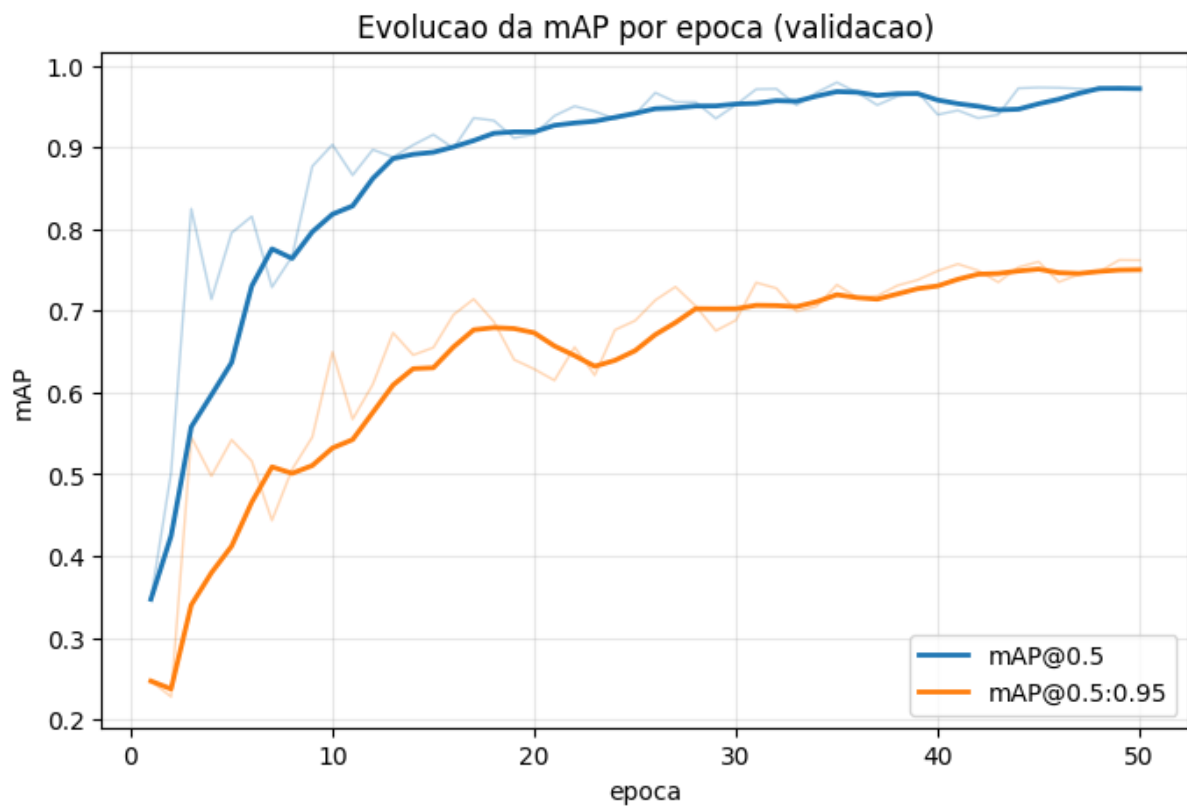
Figura 6 - Gráfico da métrica mAP por época
