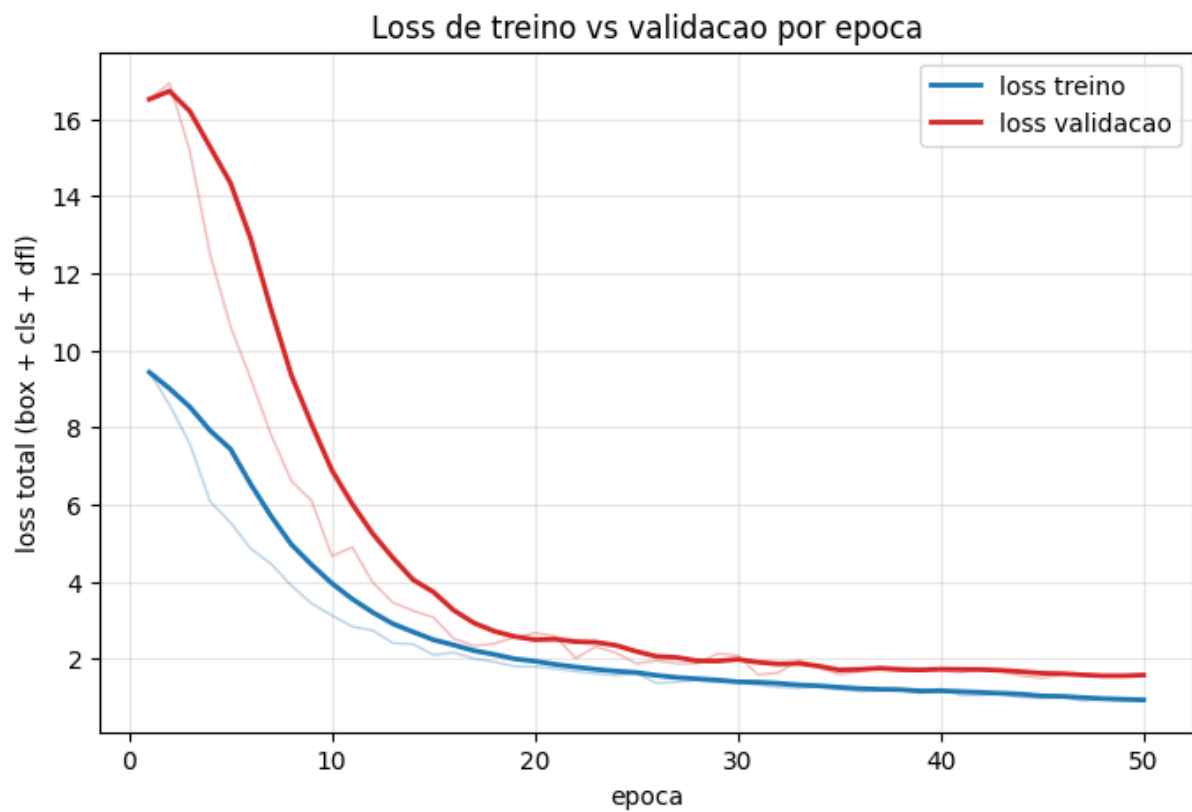
Figura 5 - Gráfico de Loss por Época
